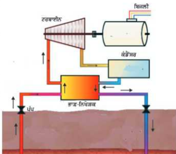
ਚਿੱਤਰ 13.5 ਭੂ-ਤਾਪ ਪਾਵਰ ਪਲਾਂਟ
