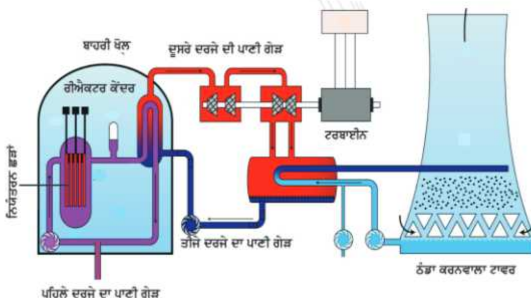
ਚਿੱਤਰ 13.7 ਨਿਊਕਲੀਅਰ ਪਾਵਰ ਪਲਾਂਟ ਦੀ ਰਚਨਾ
